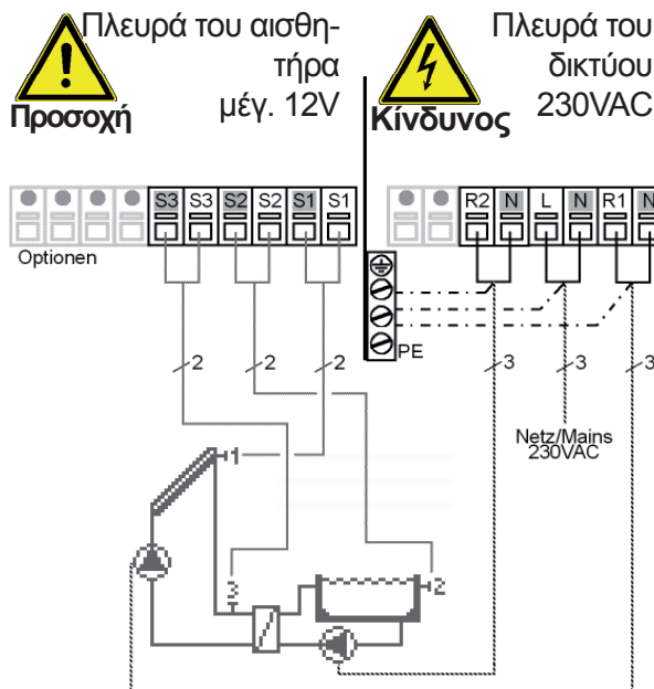
Εικ. 3.2.13 "Ηλιακό σύστημα με πισίνα"
