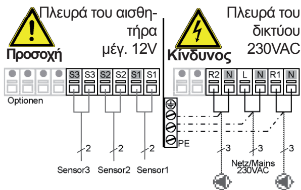
Εικ. 3.2.15 "Ρυθμιστής Δθ πολλών χρήσεων"
